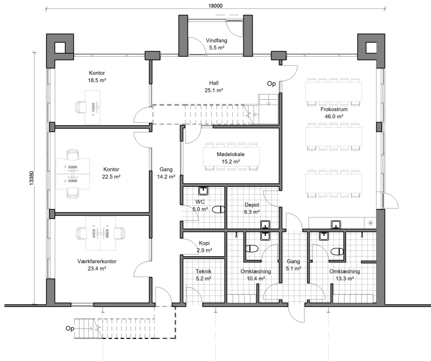
Grundplan
